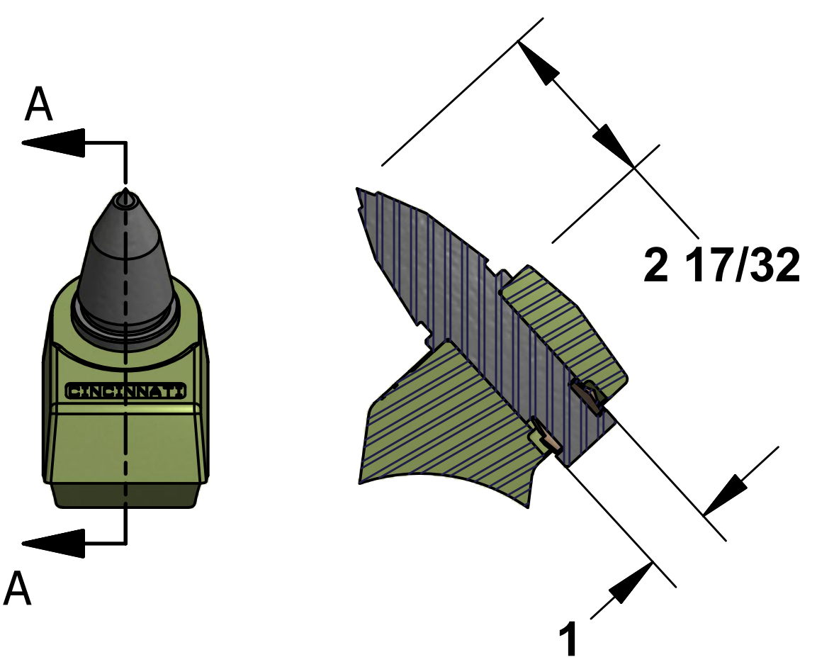
SECTION A-A
